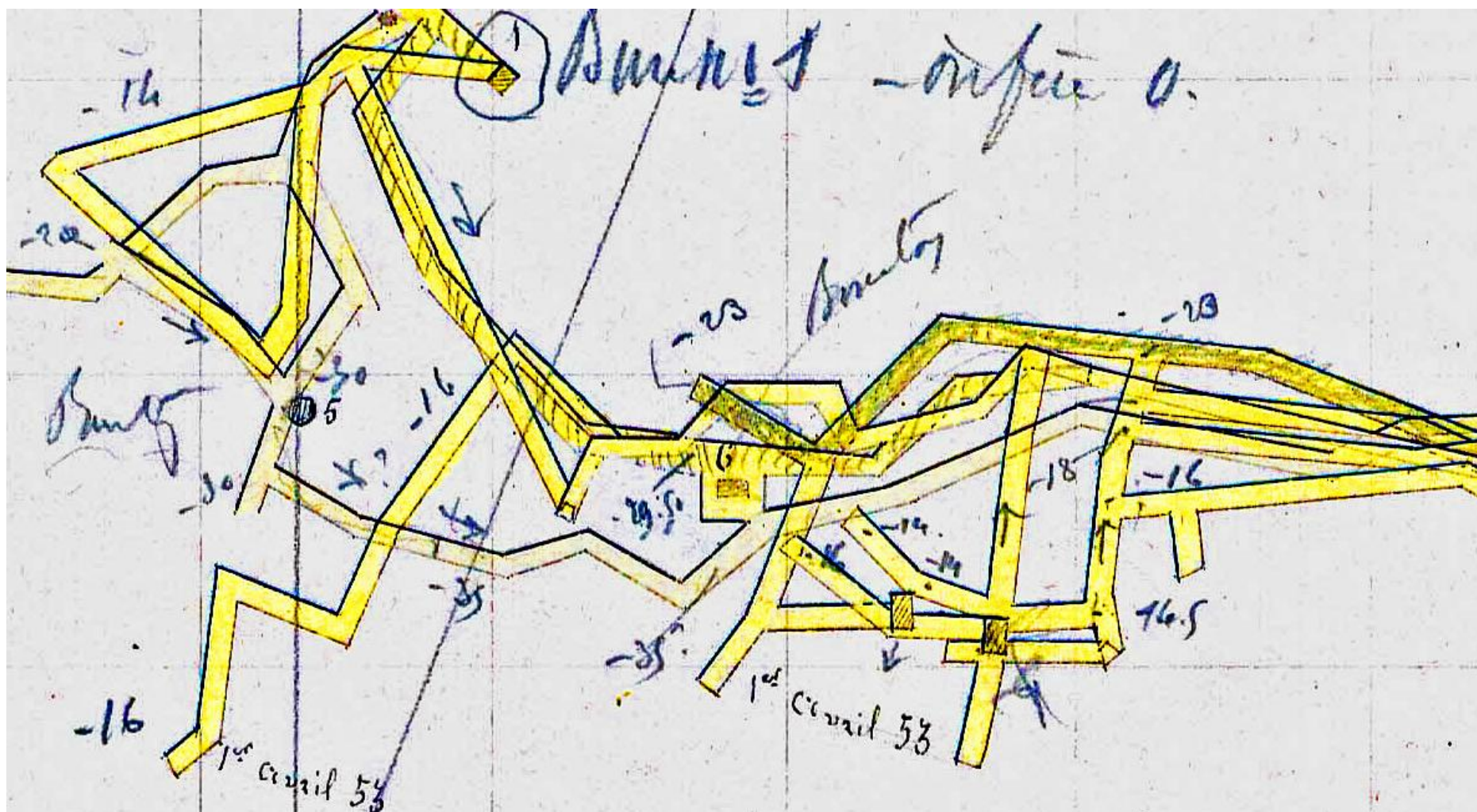
Détail des galeries entre 14 m et 35 m à proximité du bure 1 (repère de niveau). Les dates d'arrêt des travaux de prospection sont indiquées (1 er avril 1853). Les boustays principaux 5 et 6 sont repérés.
